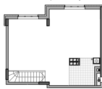
■ Схема перепланування. 10 поверх. М 1:200
