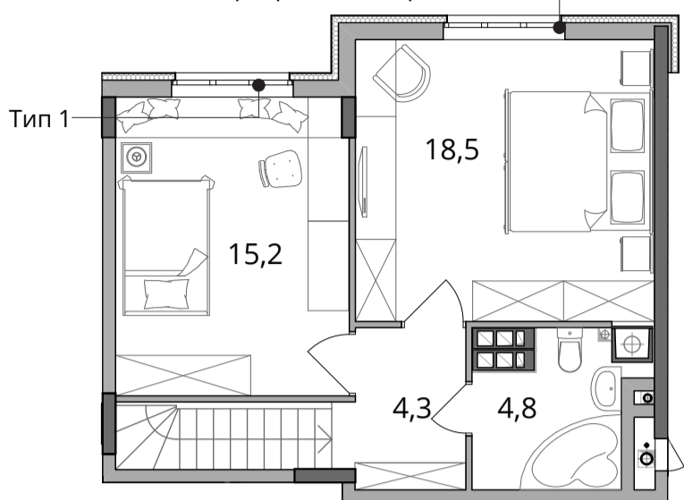
■ План квартири. 10 поверх. М 1:100
