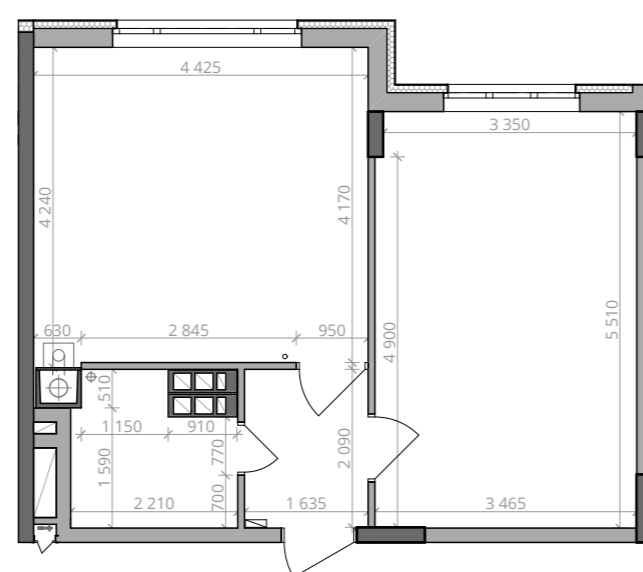
■ Габарити приміщень. М 1:100
