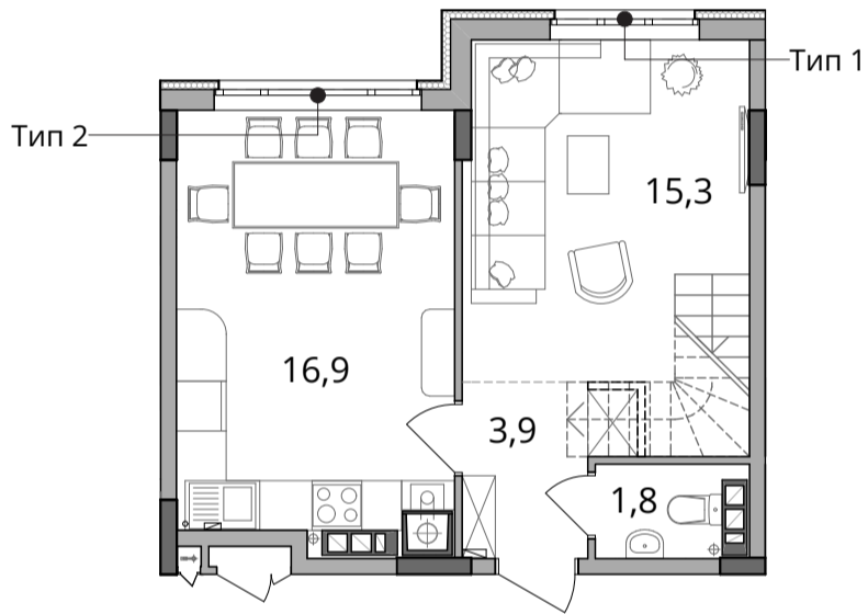
■ План квартири. 9 поверх. М 1:100
