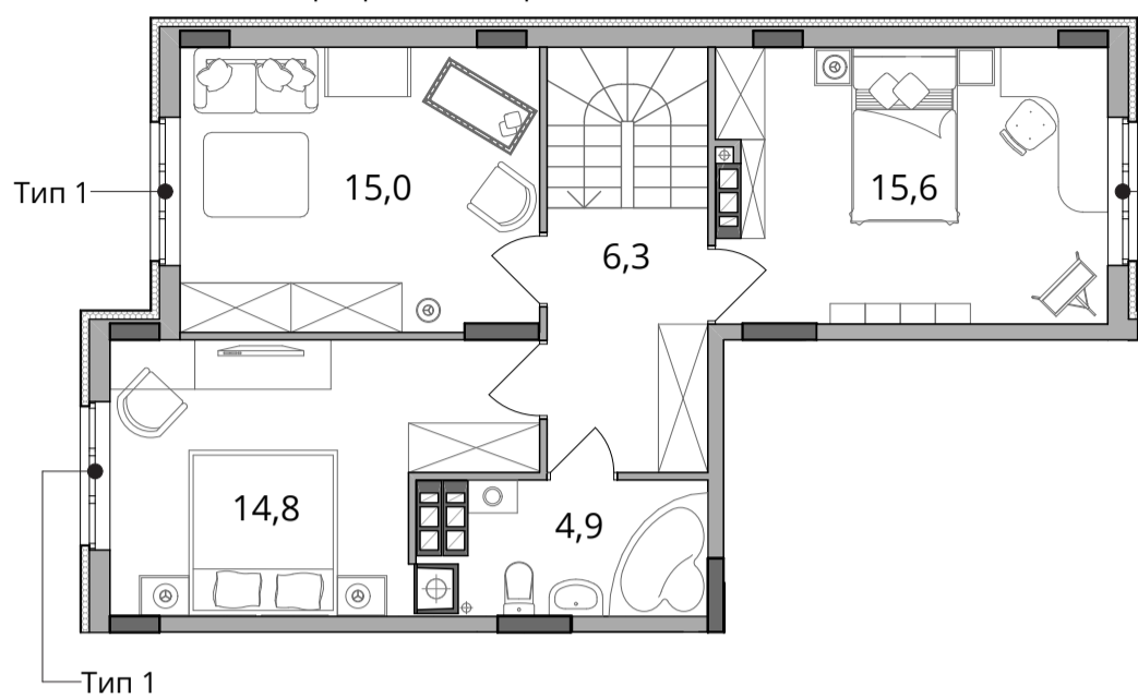
■ План квартири. 10 поверх. М 1:100
