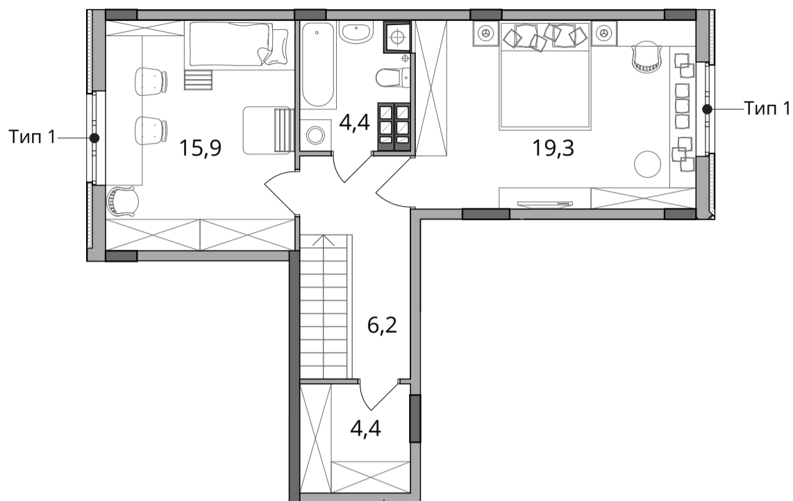
■ План квартири. 10 поверх. М 1:100
