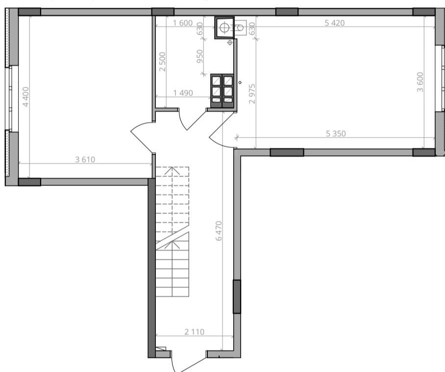
■ Габарити приміщень. 9 поверх. М 1:100
