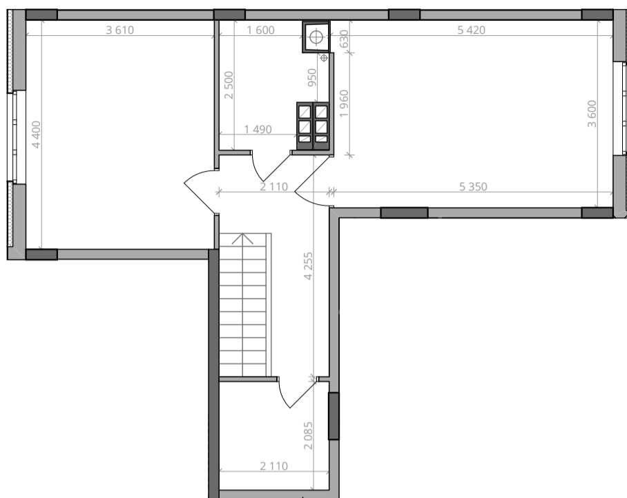
■ Габарити приміщень. 10 поверх. М 1:100
