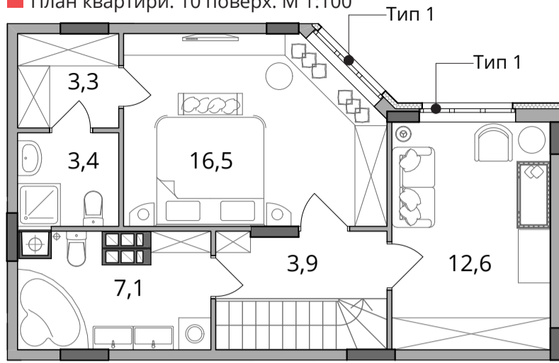
■ План квартири. 10 поверх. М 1:100
