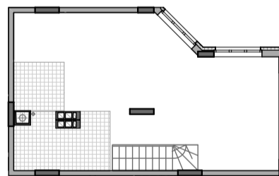
■ Схема перепланування. 10 поверх. М 1:200
