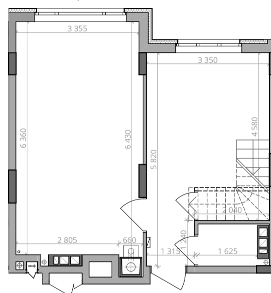
■ Габарити приміщень. 9 поверх. М 1:100
