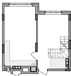
■ Схема перепланування. 9 поверх. М 1:200
