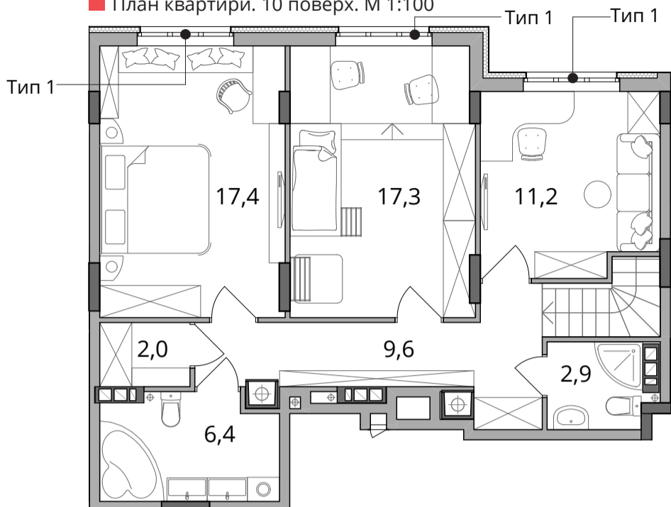
■ План квартири. 10 поверх. М 1:100
