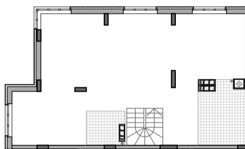
■ Схема перепланування. 10 поверх. М 1:200
