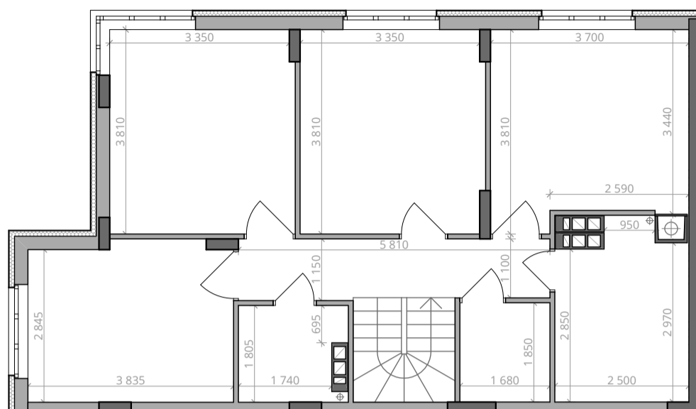
■ Габарити приміщень. 10 поверх. М 1:100
