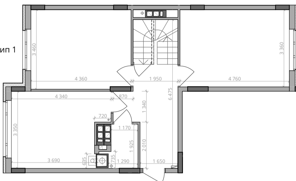
■ Габарити приміщень. 10 поверх. М 1:100
