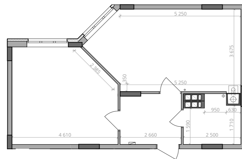
■ Габарити приміщень. М 1:100
