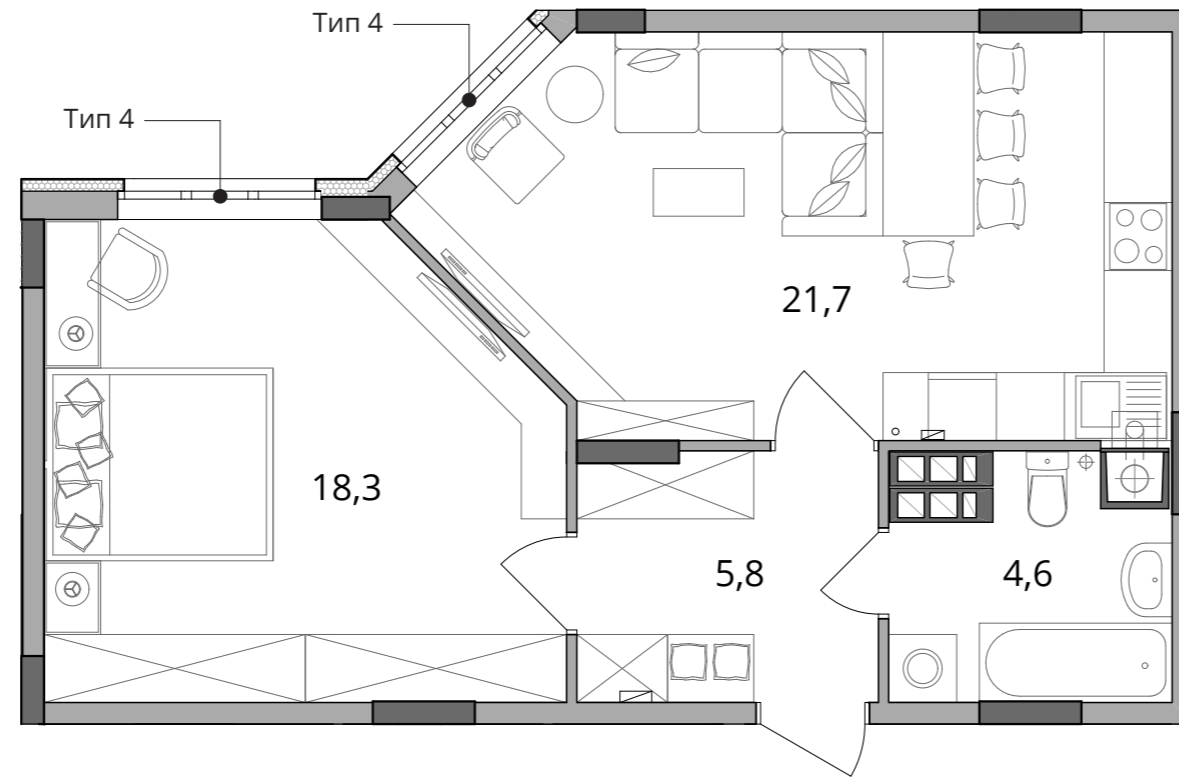
■ План квартири. М 1:75
