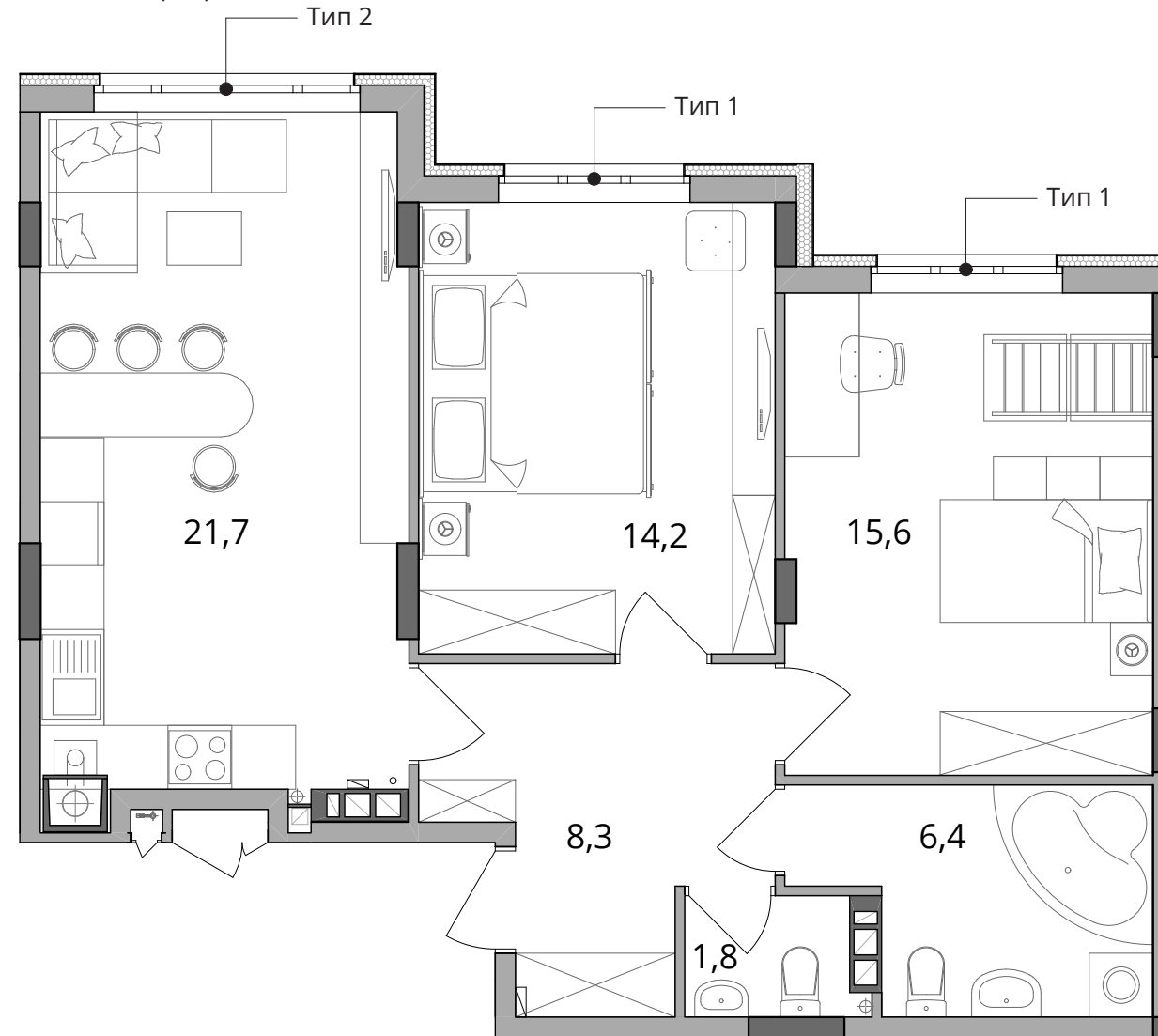
■ План квартири. М 1:75
