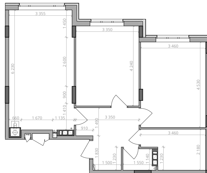
■ Габарити приміщень. М 1:100
