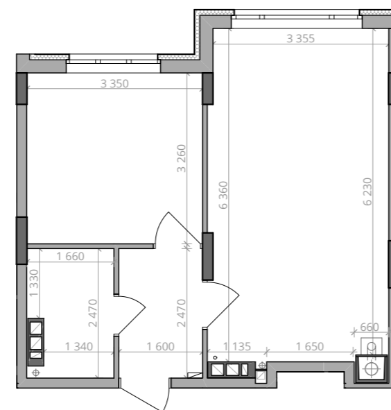
■ Габарити приміщень. М 1:100
