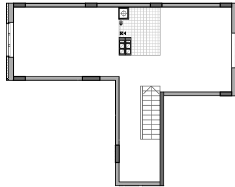
■ Схема перепланування. 10 поверх. М 1:200
