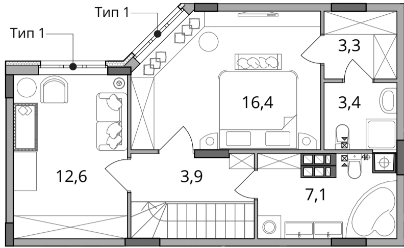
■ План квартири. 10 поверх. М 1:100
