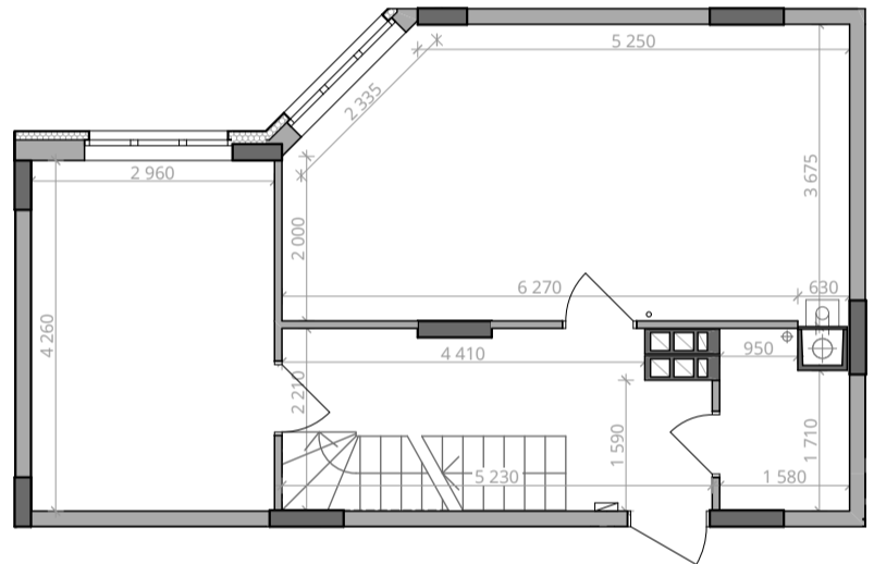
■ Габарити приміщень. 9 поверх. М 1:100
