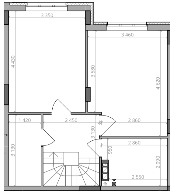
■ Габарити приміщень. 9 поверх. М 1:100
