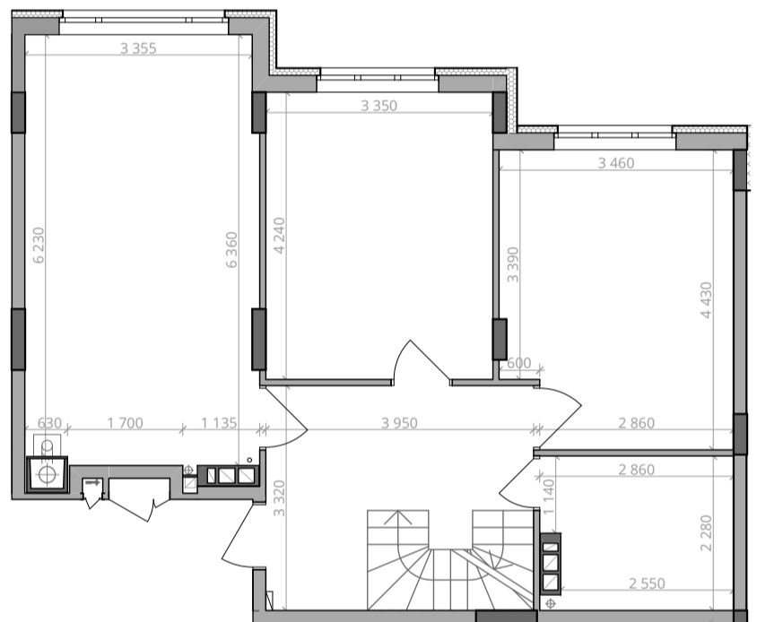
■ Схема перепланування. 10 поверх. М 1:200
