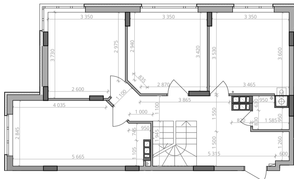
■ Габарити приміщень. 9 поверх. М 1:100
