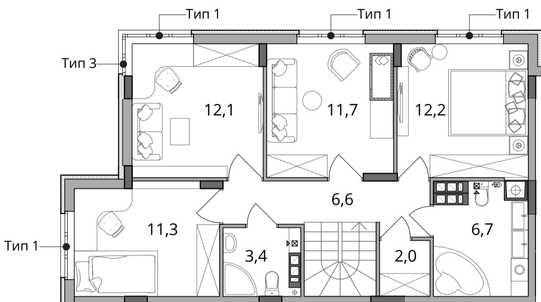
■ План квартири. 10 поверх. М 1:100
