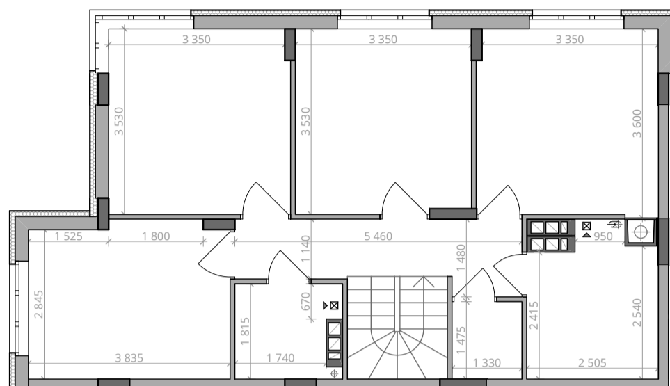
■ Габарити приміщень. 10 поверх. М 1:100
