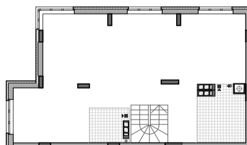
■ Схема перепланування. 10 поверх. М 1:200
