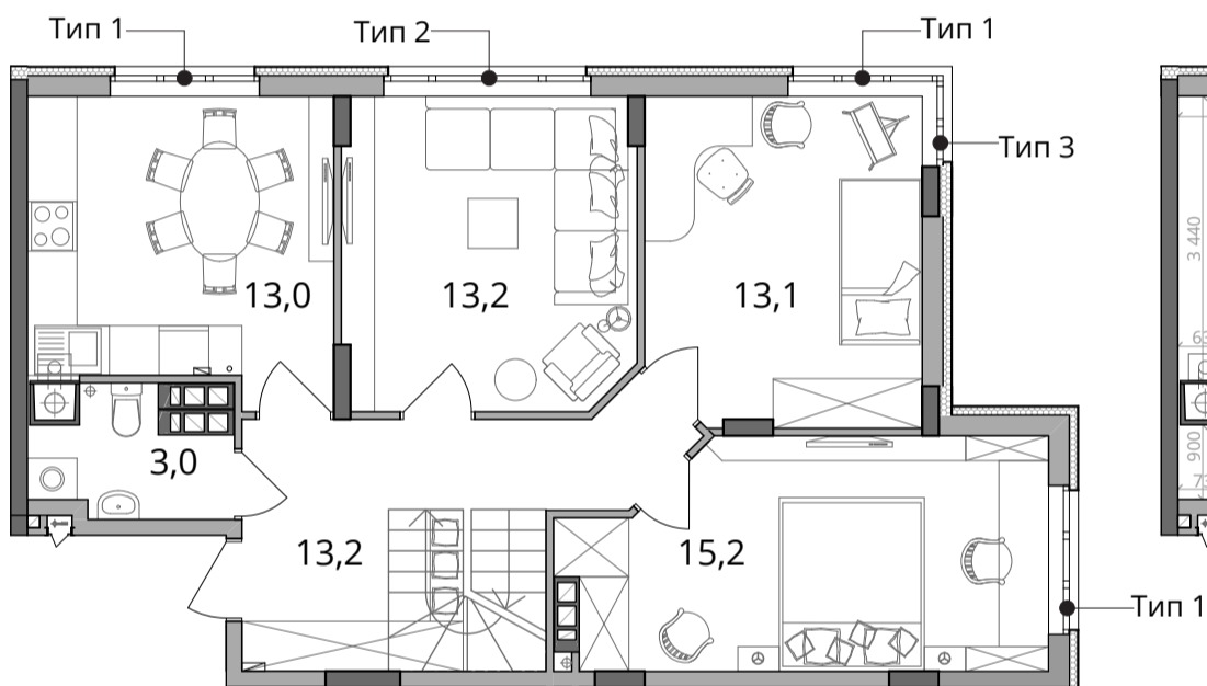
■ План квартири. 9 поверх. М 1:100
