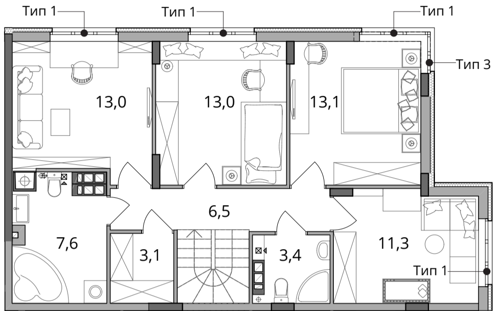
■ План квартири. 10 поверх. М 1:100
