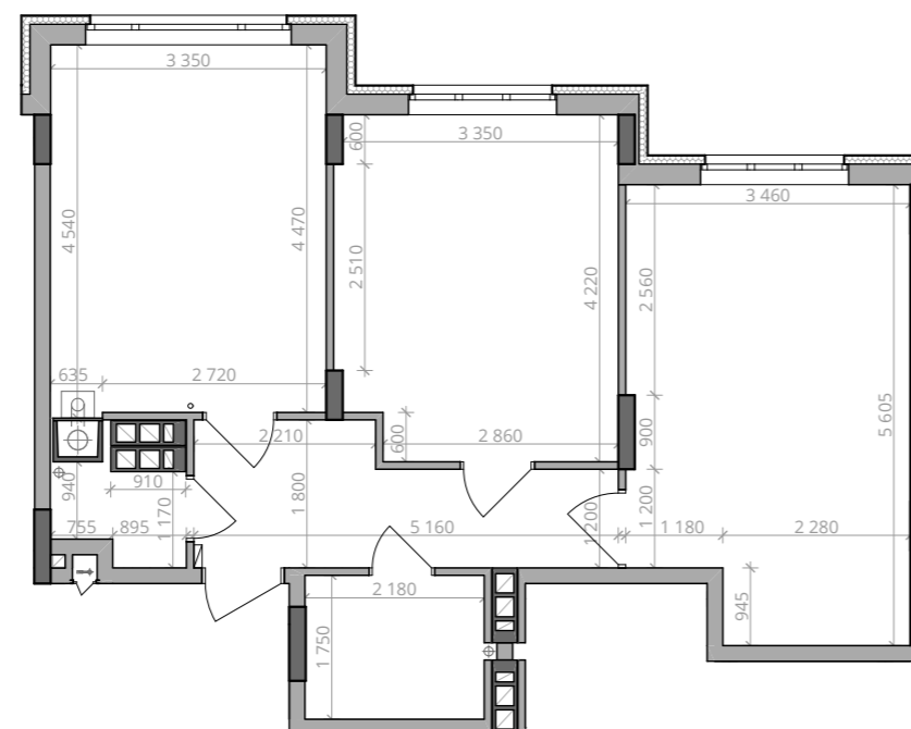
■ Габарити приміщень. М 1:100
