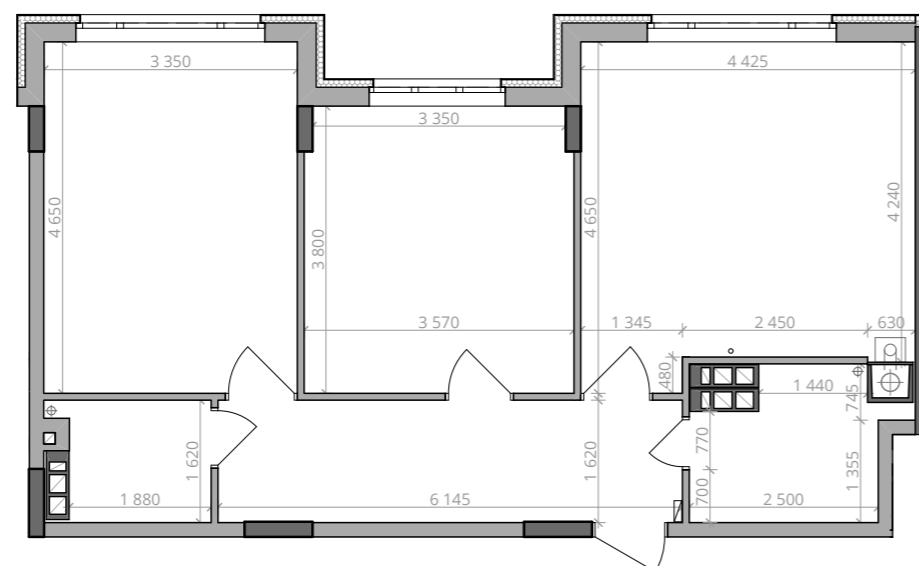
■ Габарити приміщень. М 1:100
