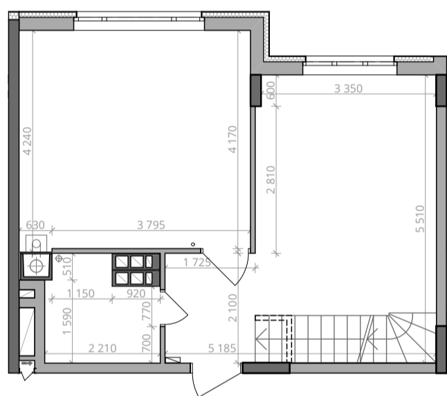
■ Габарити приміщень. 9 поверх. М 1:100
