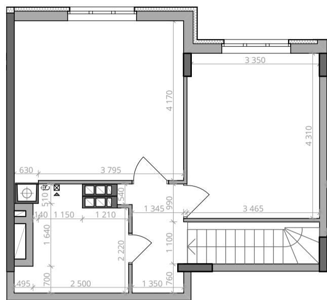
■ Габарити приміщень. 10 поверх. М 1:100
