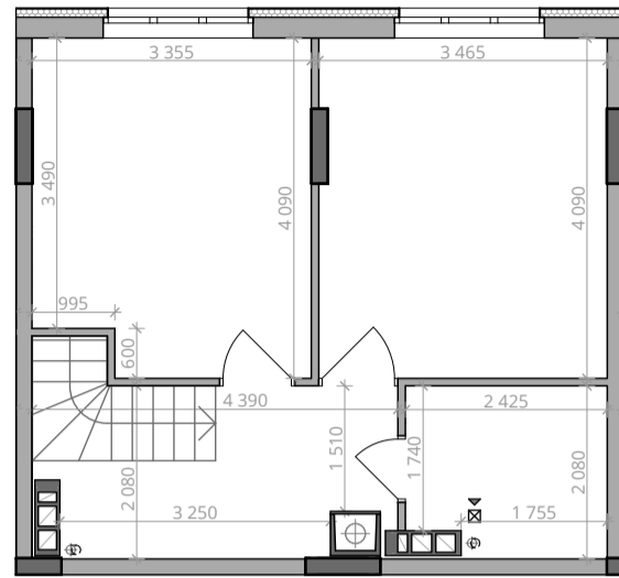
■ Габарити приміщень. 10 поверх. М 1:100
