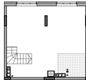
■ Схема перепланування. 10 поверх. М 1:200
