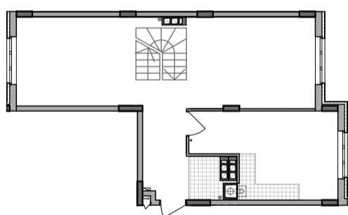
■ Схема перепланування. 9 поверх. М 1:200
