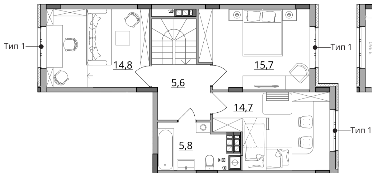
■ План квартири. 10 поверх. М 1:100
