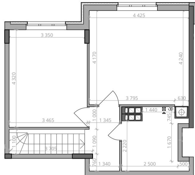
■ Габарити приміщень. 10 поверх. М 1:100
