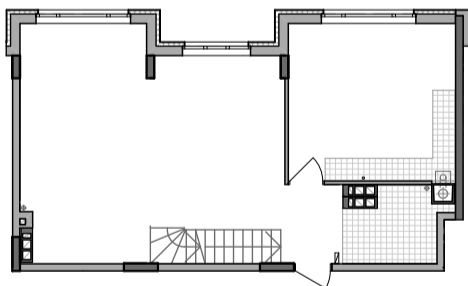
■ Схема перепланування. 9 поверх. М 1:200
