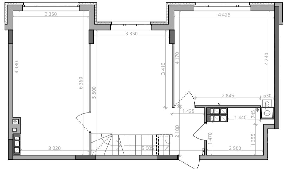
■ Габарити приміщень. 9 поверх. М 1:100
